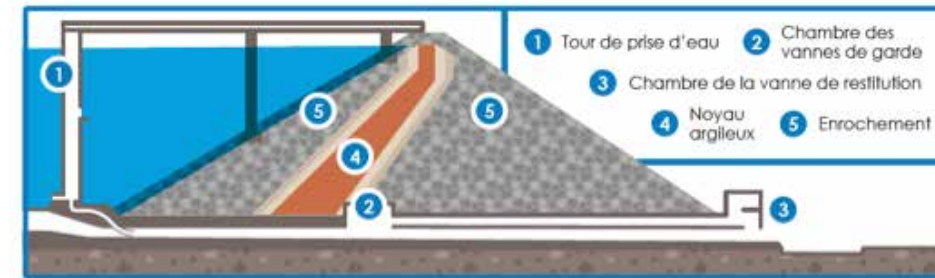
Construction de la tour d'exhaure – barrage de la Chèze
